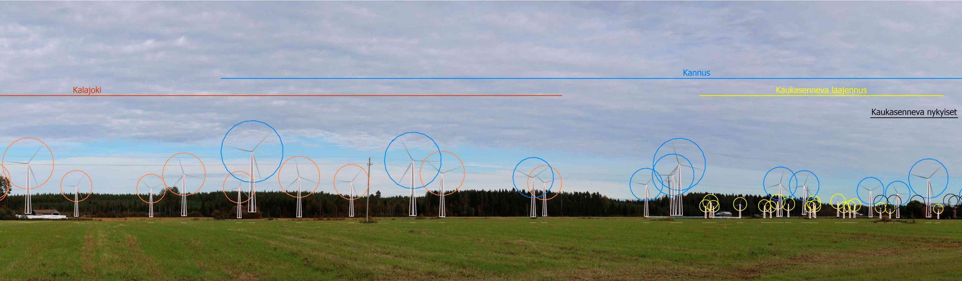
Kuvauspaikka 1 yhteisvaikutukset, Kannus, Väli-Kannus, Himangantie. Koostettu panorama, kuvattu 50 mm polttovälillä. Voimaloiden kokonaiskorkeus 295 m. Etäisyys lähimpään voimalaan noin 2,5 km.
